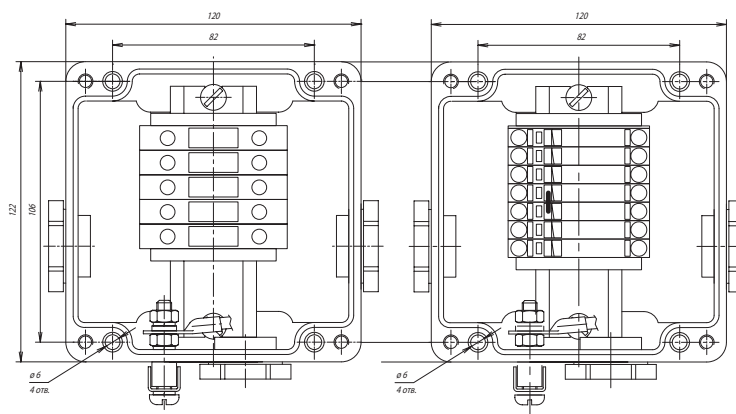
Коробка с винтовым клеммным блоком
