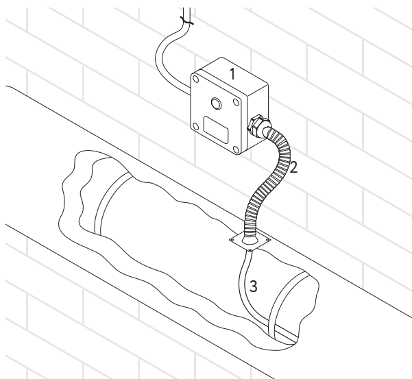
1 – соединительная коробка ВЭК 122.C 2 – рукав (защитная трубка) 3 – нагревательная секция (кабель)
